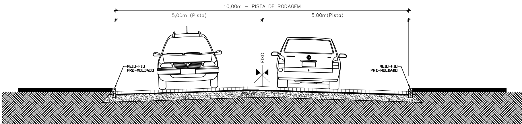
SEÇÃO TIPO DE BLOCO INTERTRAVADO - TRAVESSA GUAÍBA
